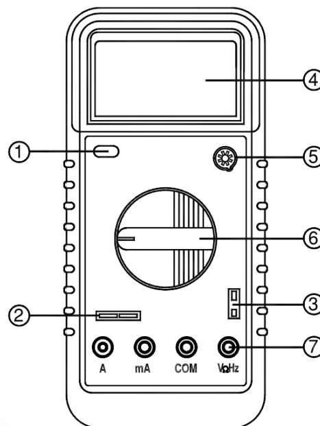
Рисунок 1. Схема мультиметра
