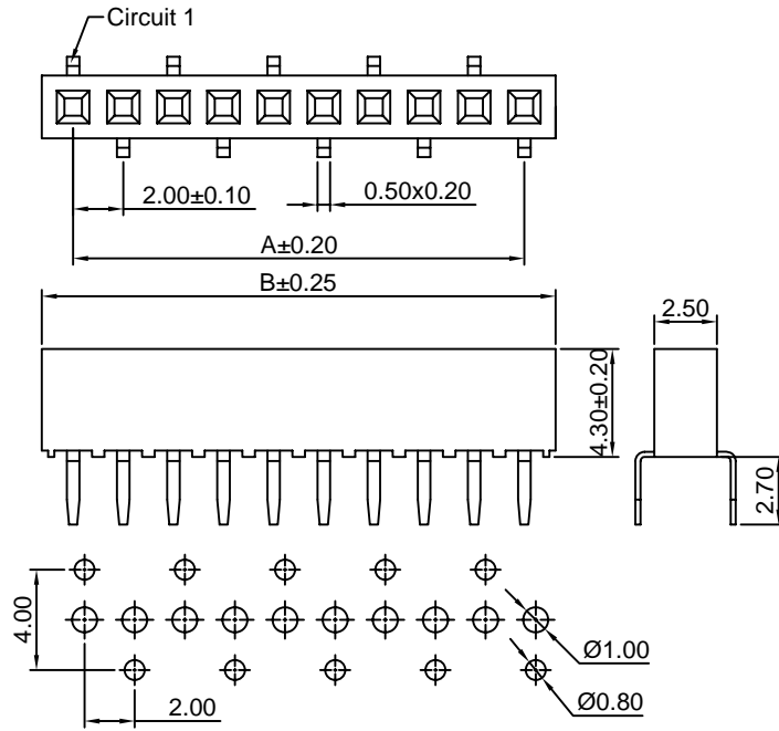
P.C.B LAYOUT
