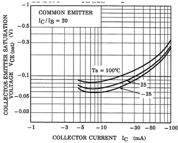
Fig. 10.19 RN2401 V_{CE(sat)} - I_C
