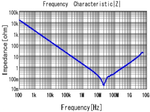
GCM21BR71H104KA37 |Z| DCOV, 25degC
