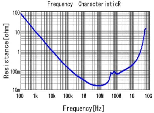
GCM21BR71H104KA37 R DCOV, 25degC
