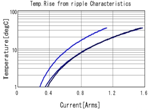
GCM21BR71H104KA37 Temp. rise ■ 400kHz ■ 800kHz ■ 1MHz
