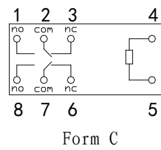
接线图
