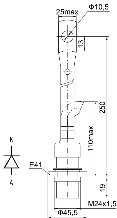
Рис. 12. Габаритные и установочные размеры
