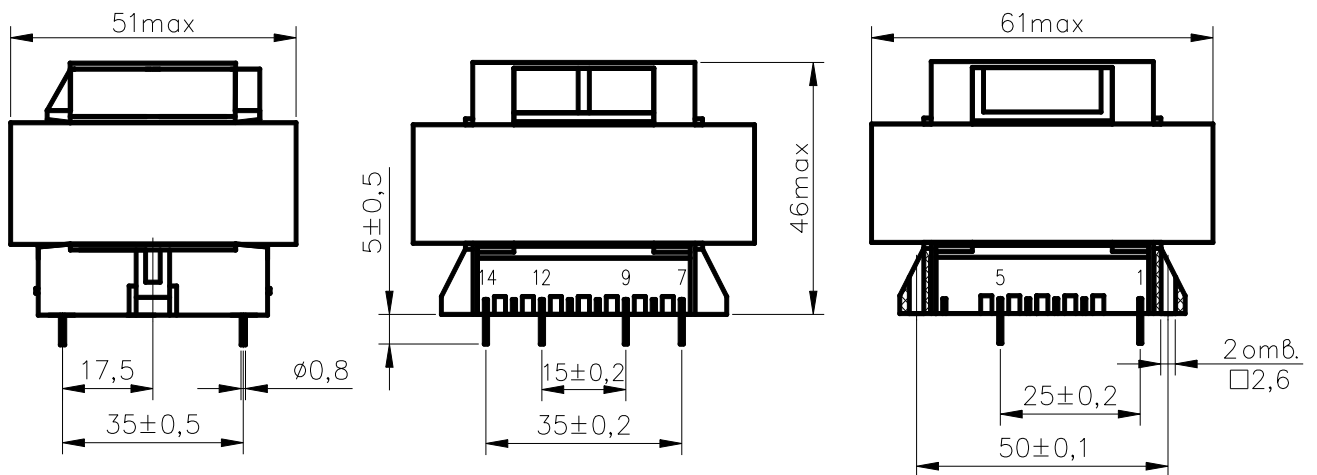
Общий вид трансформатора
