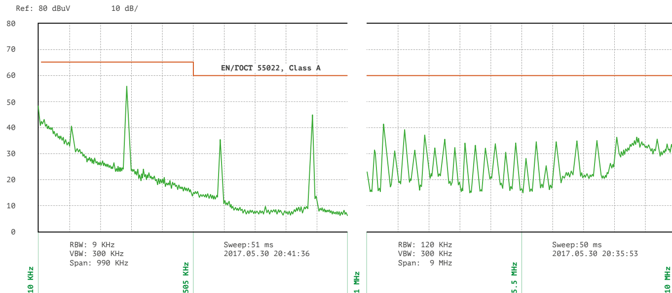
Рис. 7. Спектрограмма радиопомех VDV12 с типовой схемой подключения.
