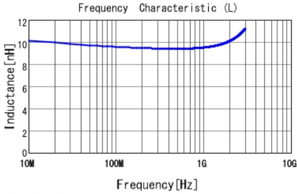
■ LQW15AN9N5G00 L
