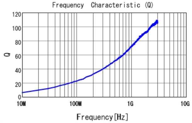
■ LQW15AN9N5G00 Q
