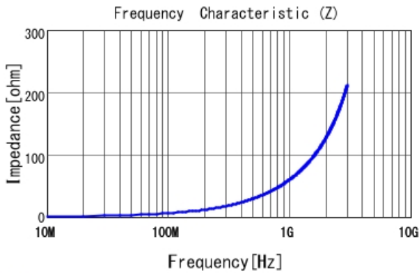
■ LQW15AN9N5G00 |Z|
