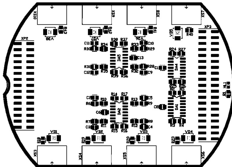
Рис. 1.2 Расположение элементов платы AI board
