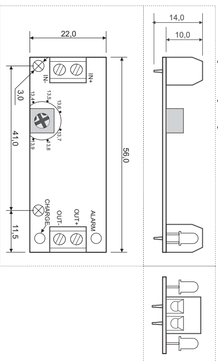
Рис. 2. Габаритные размеры
