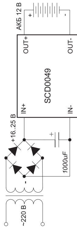
Рис. 1. Схема включения
