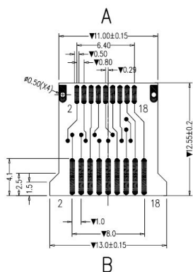
Dimensions : Millimetres
