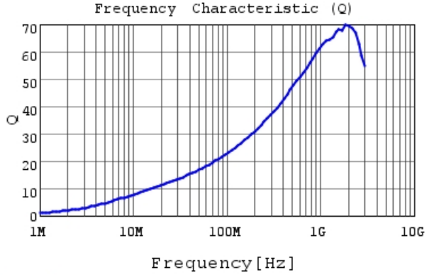
LQW15AN22NG8Z Q
