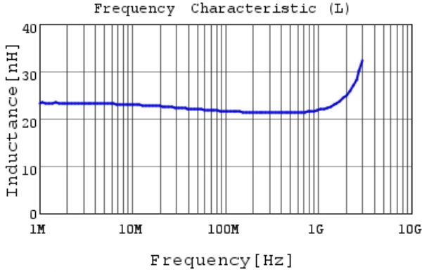
LQW15AN22NG8Z L
