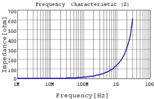
LQW15AN22NG8Z |Z|
