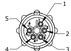
WIRING VIEW W18982-5SG-P-5XX
