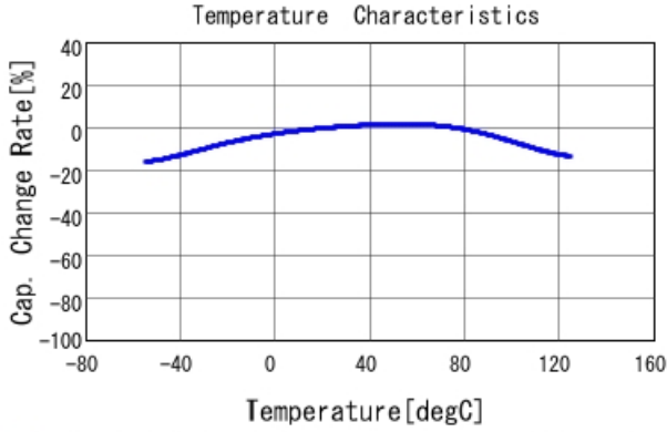
■ GRM033C71C104ME14 C-Temp. capchange, DCO. 0V, ACO. 2V rm
