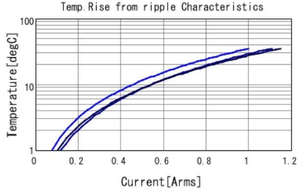
GRM033C71C104ME14 Temp. rise ■ 400kHz ■ 800kHz ■ 1MHz
