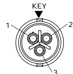
WIRING END W6382-3SG-P-3XX
