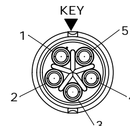
WIRING END W6382-5SG-P-3XX
