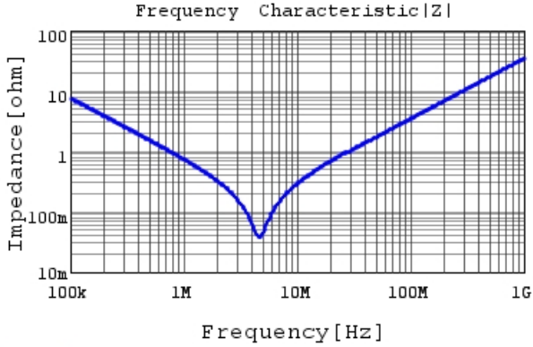
RDER72E224K3M1H03A |Z| DCOV, 25degC
