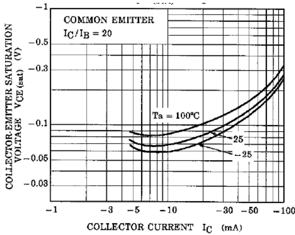
Fig. 10.19 RN2301 V_{CE(sat)}-I_C
