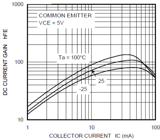
Fig. 10.11 RN1114 h_{FE}-I_C
