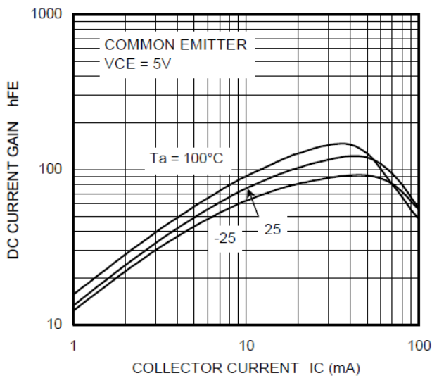
Fig. 10.13 RN1116 h_{FE}-I_C
