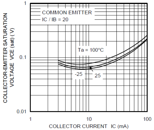
Fig. 10.17 RN1115 V_{CE(sat)}-I_C
