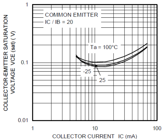
Fig. 10.19 RN1117 V_{CE(sat)}-I_C
