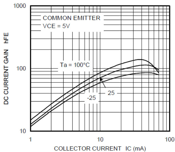
Fig. 10.13 RN1116 h_{FE}-I_C
