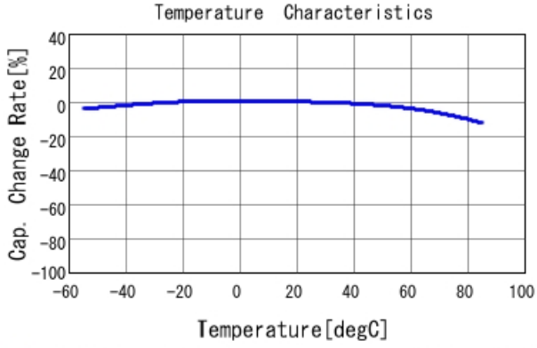
■ GRM21BR61A226ME51 C-Temp. capchange, DCO. 0V, ACO. 5Vrm
