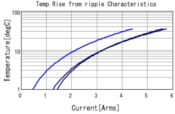
GRM21BR61A226ME51 Temp. rise ■ 80kHz ■ 400kHz ■ 800kHz
