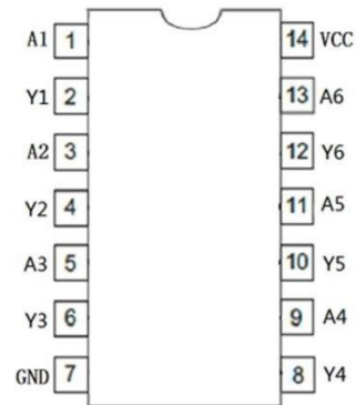
图 3、引脚排列图
