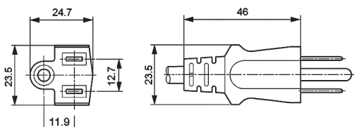
NEMA5-15
