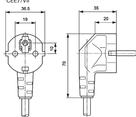
CEE7/VII
