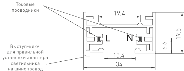
Рис. 1. Чертеж и конструкция шинопровода.
