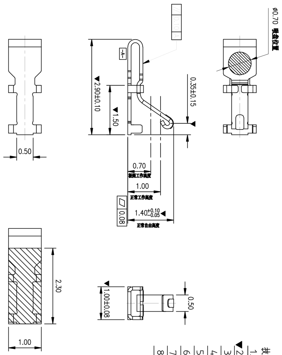
焊盘尺寸
