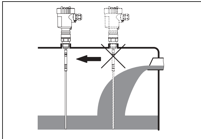
Fig. 2: Lateral load
