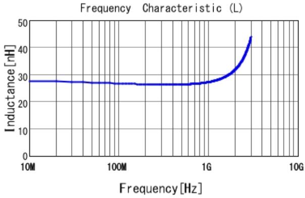
■ LQW15AN27NJ00 L
