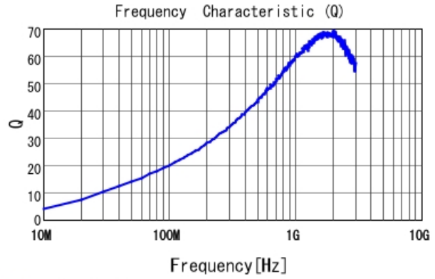
■ LQW15AN27NJ00 Q
