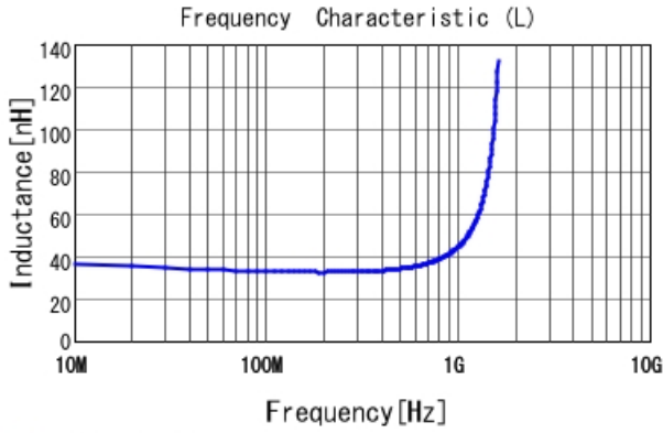
■ LQG18HN33NJ00 L
