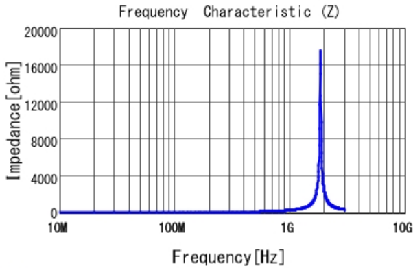
■ LQG18HN33NJ00 |Z|
