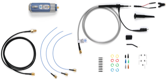
Пробник R&S®RT-ZPR20 поставляется с большим набором стандартных принадлежностей для всевозможных типов подключений.
