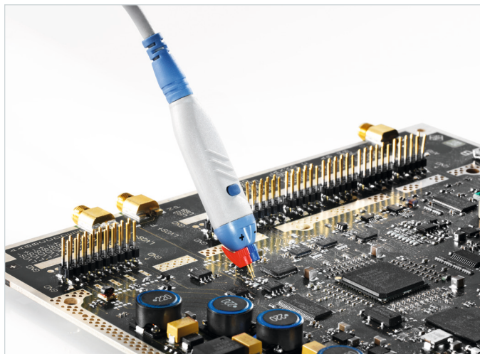
Компактный активный широкополосный пробник R&S®RT-ZD40.
