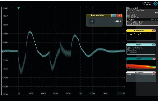
Возможность точной проверки уровня постоянного тока и характеристики нагрузки по питанию во время инициализации памяти DDR3 с помощью функции R&S®ProbeMeter и гибких математических функций осциллографа R&S®RTO.
