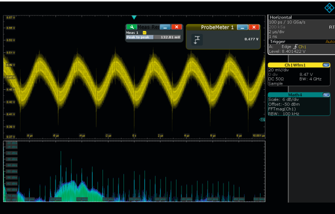
Высокая полоса пропускания пробника R&S®RT-ZPR20 позволяет захватывать даже высокочастотные шумовые составляющие, которые можно легко проанализировать с помощью функции спектрального анализа осциллографа R&S®RTO.
