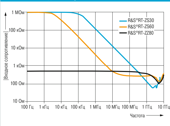
Зависимость входного сопротивления от частоты
