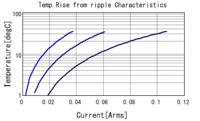
GRM188R72E152KW07 Temp. rise — 30kHz — 100kHz
