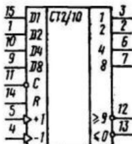
Условное графическое изображение K155IE6, KM155IE6
