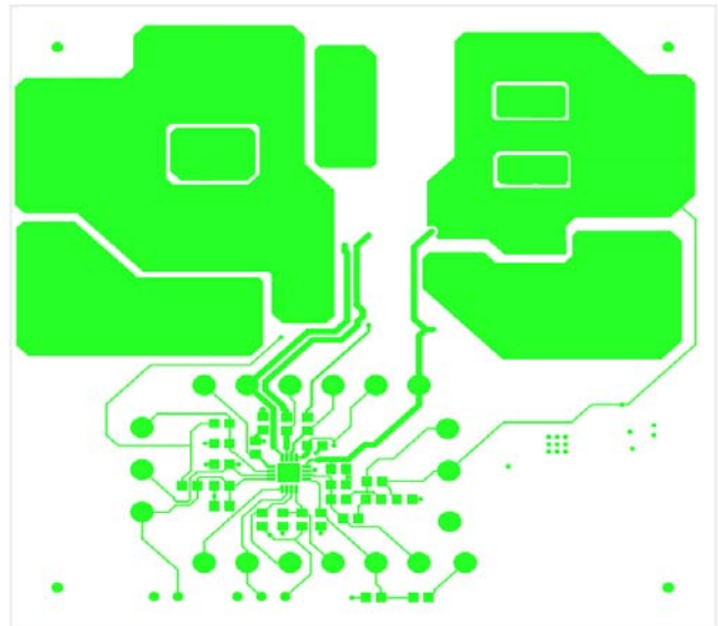
FIGURE 22. TOP LAYER
