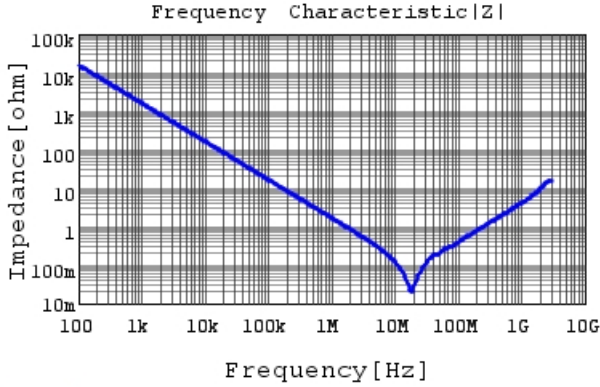
GRM32DR72H104KW10 |Z| DCOV,25degC
