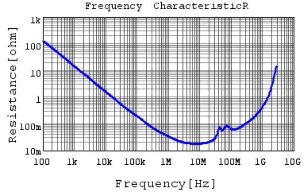
GRM32DR72H104KW10 R DCOV,25degC
