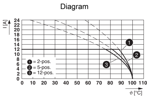
Type: GFKC 2,5/...-ST-7,62 with GMSTBA 2,5/...-G-7,62
