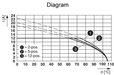
Type: GFKC 2,5/...-ST-7,62 with GMSTBV 2,5/...-G-7,62
