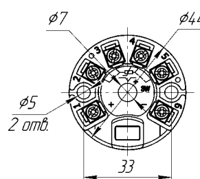
Рисунок 3.1 – Габаритный чертеж
