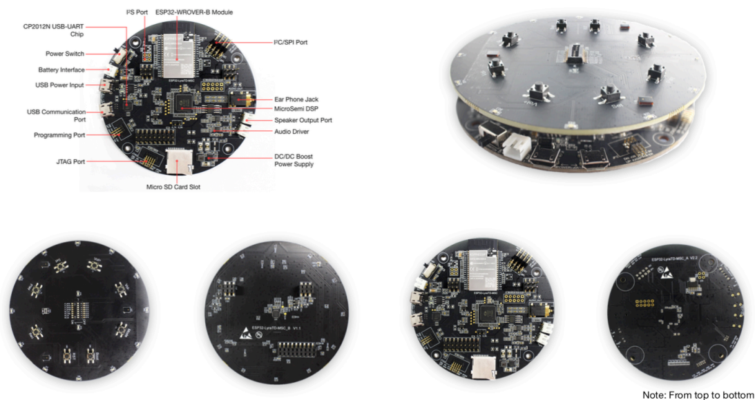
Figure 1-1. ESP32-LyraTD-MSC
