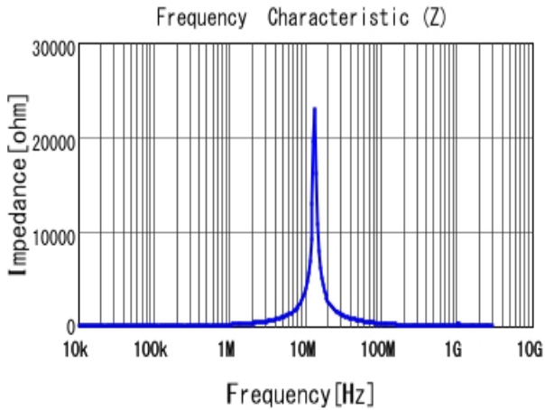
■ 1255AY-330M |Z|
