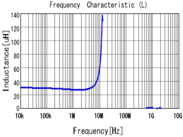
■ 1255AY-330M L
