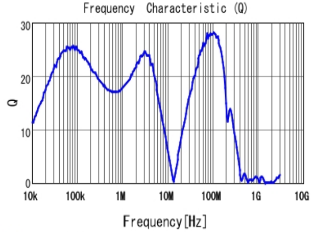
■ 1255AY-330M Q
