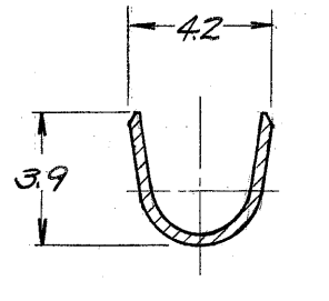
断面 C-C
