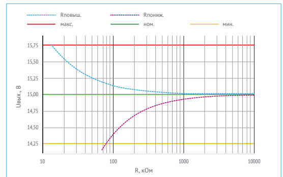
Рис. 5 (е). График зависимости для VDR160[...]15.
