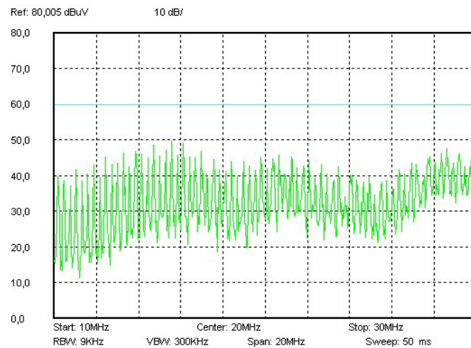
Рис. 11 (б). Спектрограмма 10–30 MHz.
