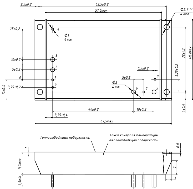
Рис. 12. Исполнение в усиленном корпусе с фланцами.
