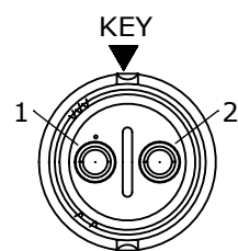
WIRING END W6382-2SG-P-3XX
