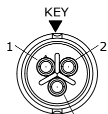
WIRING END W6382-3SG-P-3XX
