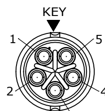
WIRING END W6382-5SG-P-3XX
