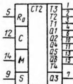
Условное графическое обозначение К176ИЕ18
