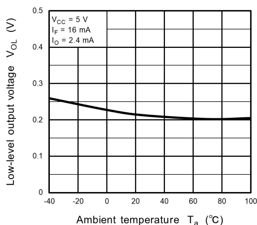
Fig. 13.2.10 V_{OL} - T_a
