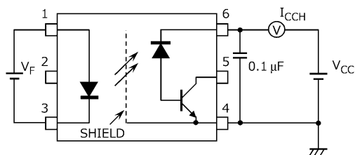
Fig. 13.1.3 I_{CCH} Test Circuit
