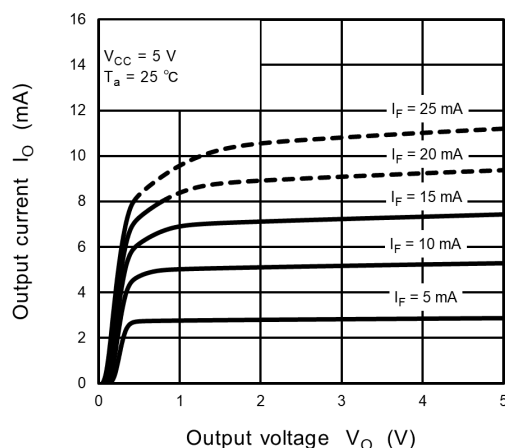
Fig. 13.2.8 I_O - V_O
