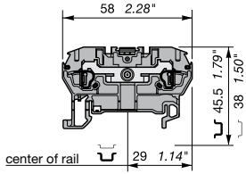
D 2,5/5.2L
