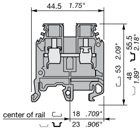
M 10/10
