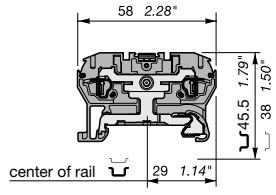
D 2,5/5.P.2L
