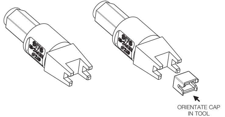
UNIVERSAL HANDLE 06 7000 7730 01 000
