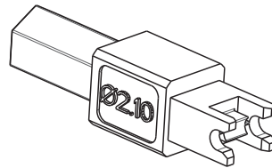
2.1 WIRE (18-20 AWG) 06-9176-7019-01-000 06-9176-7020-01-000
