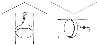
Рис. 2. Пример монтажа
