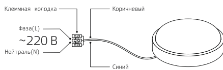
Рис. 1. Схема подключения светильника к электросети 220 В
