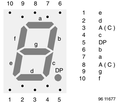
Fig. 18 - TDS.11..
