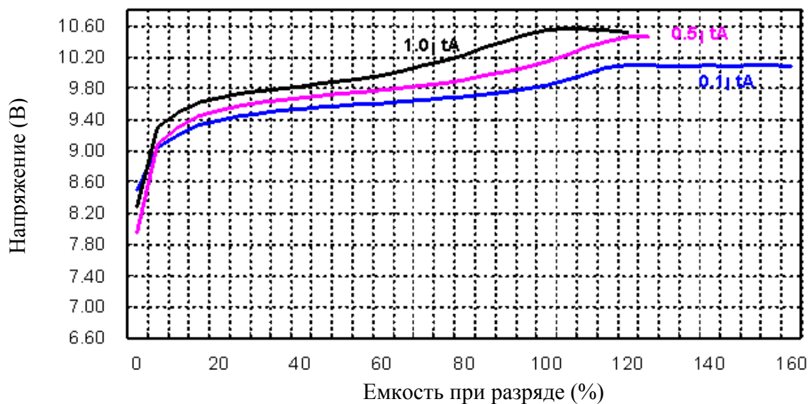
Напряжение при разряде. Температура 20С°.
