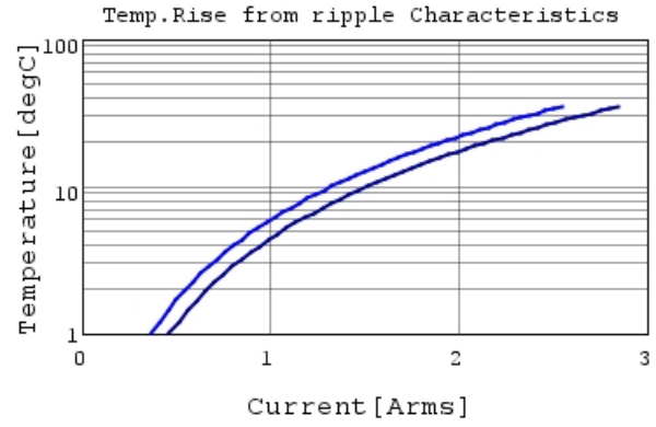
GCM155C71A105KE38 Temp.rise — 500kHz
