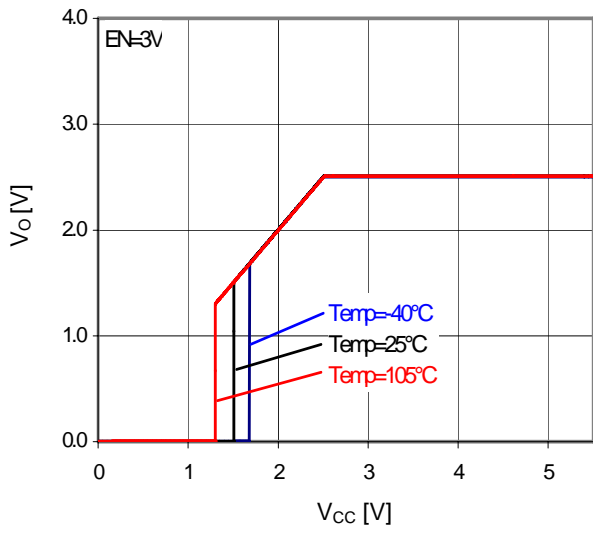
Figure 27. Vcc-Vo (Io=0mA)
