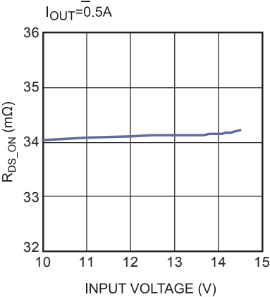
R_{DS\_ON} vs. Input Voltage
